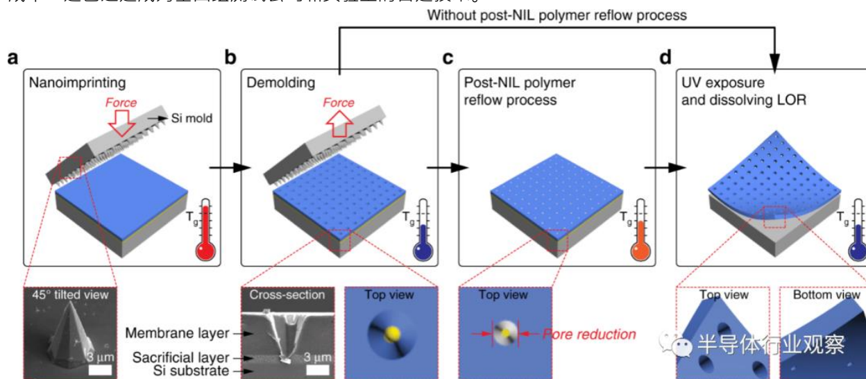
图 5：通过 NIL 和聚合物回流在独立聚合物膜中生产穿孔纳米孔的过程
