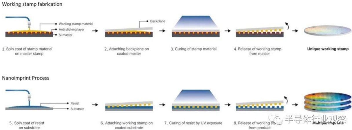
图 1：EVG 的 SmartNIL 工艺示意图，包括两个步骤——工作印章制造和压印。这两个步骤都在同一个工具中执行。
