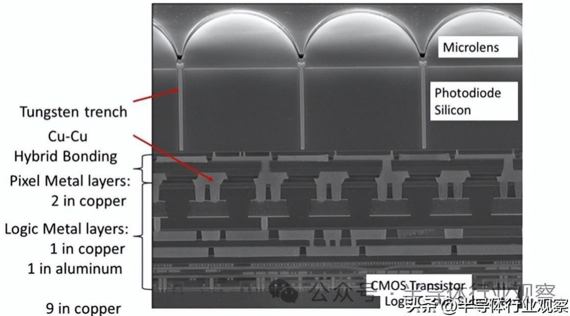
图13：在芯片间接口处使用混合键合的 NIR SPAD ToF 图像传感器的横截面
