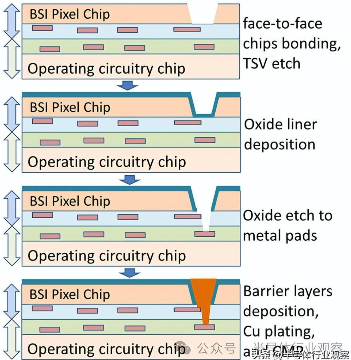
图17：用于芯片到芯片互连的后通孔 TSV 工艺流程
