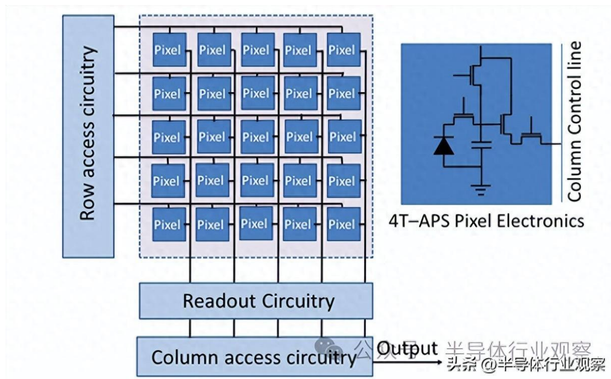
图1：成像像素阵列、电路块和典型 4 T-APS 像素电子器件的原理图
