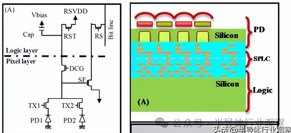
图11：像素电子分区示意图和 OmniVision 堆叠芯片像素级连接的横截面图
