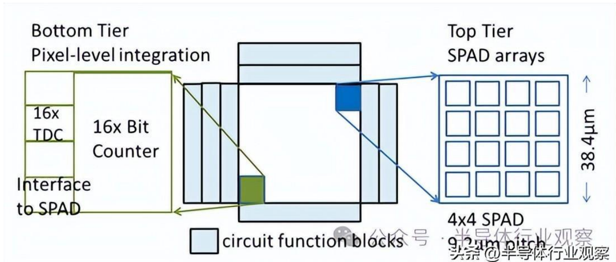
图15 : 用于 LiDAR 应用的两层 IR SPAD 传感器的芯片平面图和像素阵列
