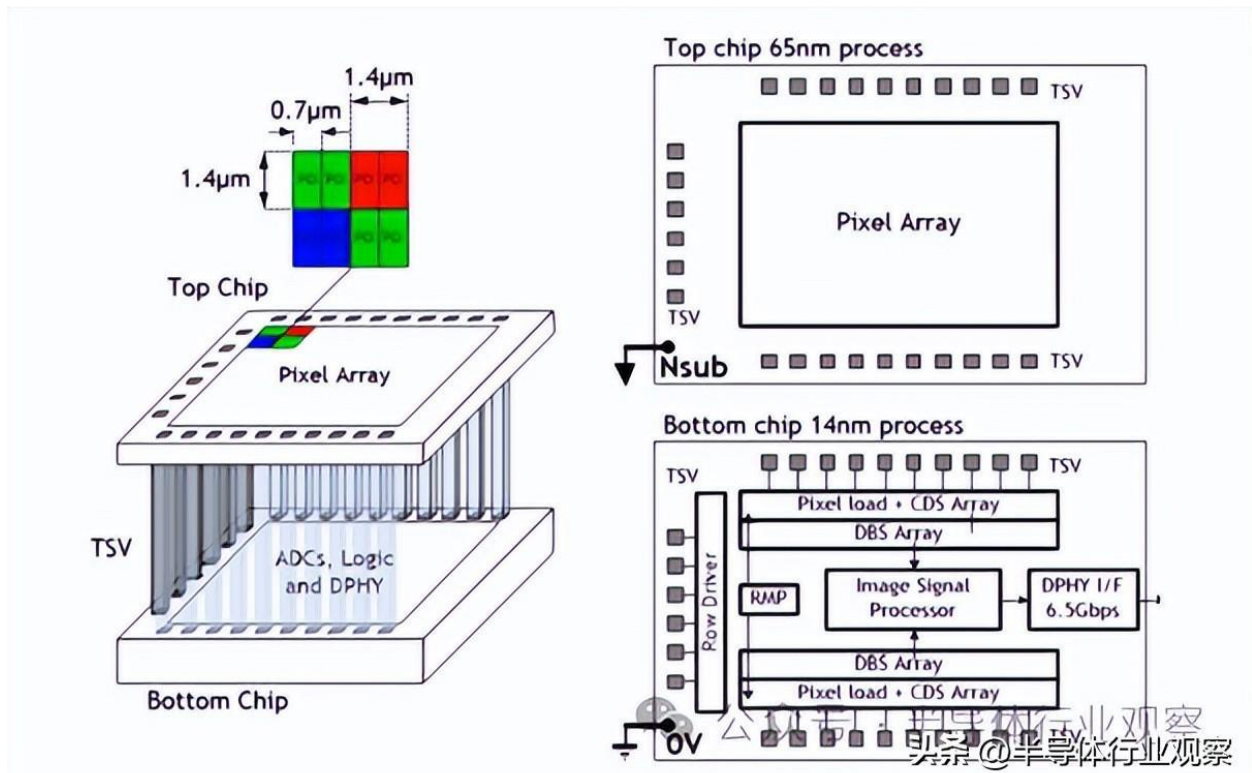
图7：采用 65 nm/14 nm 技术处理的双光电二极管堆叠芯片 BSI-CIS
