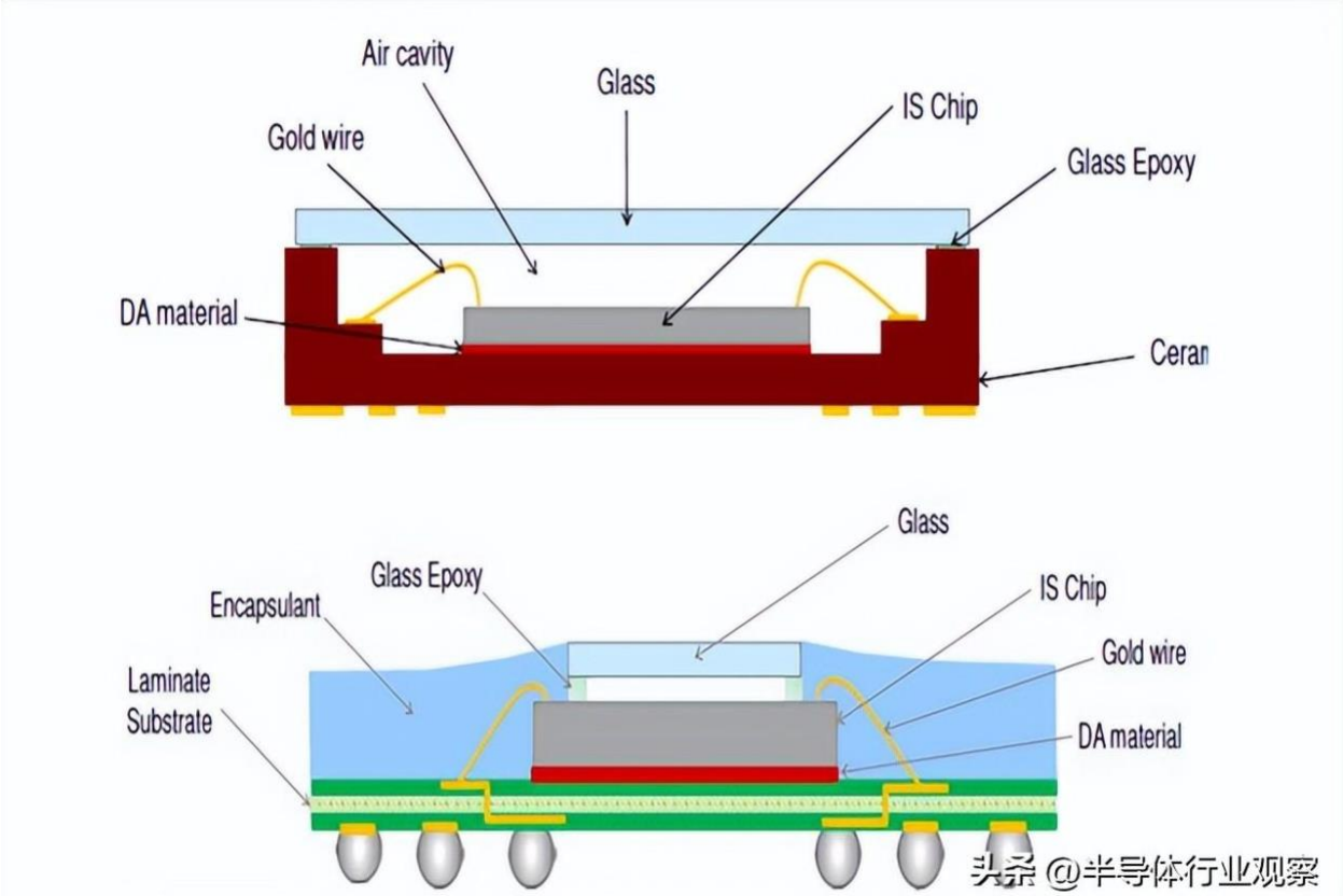
图3：顶部为陶瓷无引线芯片载体陶瓷图像传感器封装，底部为成像球栅阵列图像传感器封装的原理图
