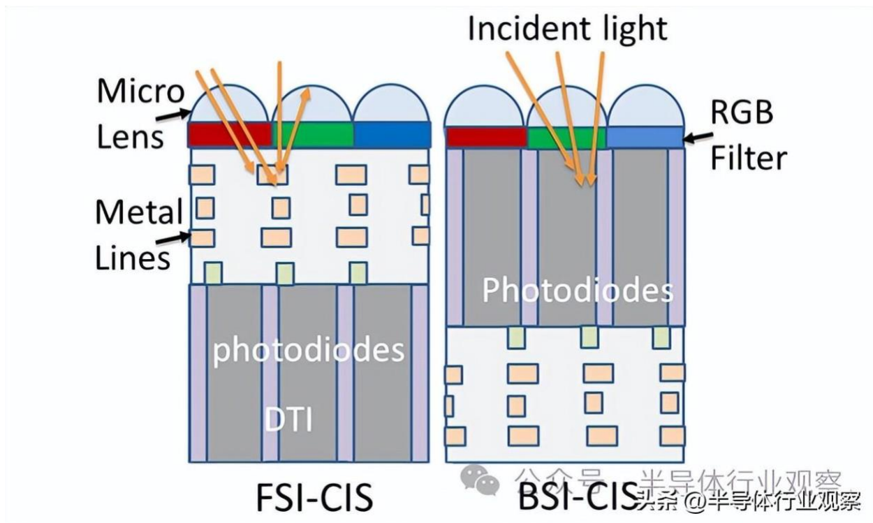
图2：正面照明传感器 (FSI-CIS) 和背面照明传感器 (BSI-CIS) 的示例原理图
