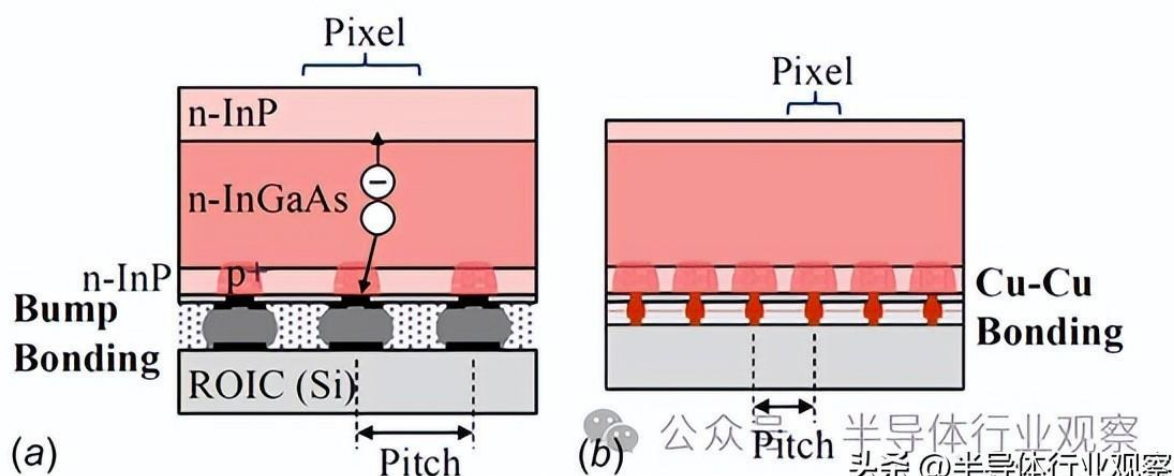
图16：使用 InP/InGaAs/InP 光电二极管通过像素级集成与硅芯片中的读出电路键合的短波长红外传感器： (a) 倒装芯片凸块和 (b) Cu-Cu 混合键合
