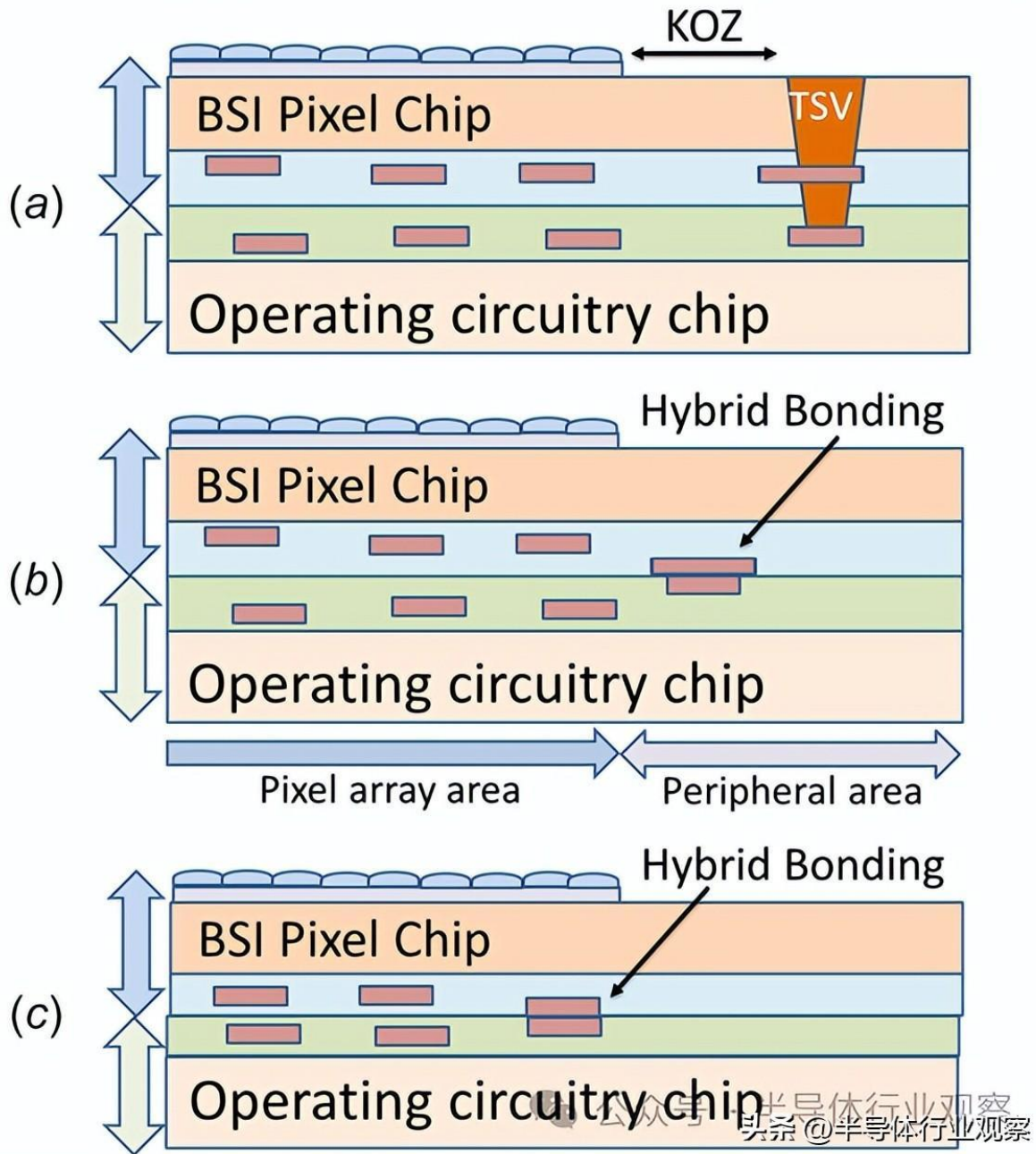
图8：芯片间键合和互连方法，其中 (a) 直接电介质键合，然后采用用于芯片间互连的后通孔 TSV，(b) 外围区域的混合键合，以及 (c) 像素阵列下的混合键合
