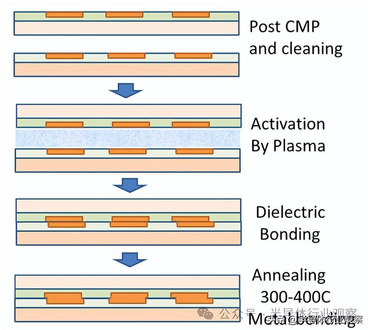
图18：直接键合互连的工艺流程
