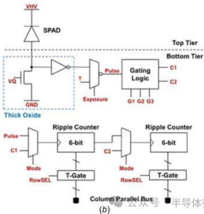
图14: 3D 堆叠式 SPAD 图像传感器示意图: (a) 通过混合键合堆叠在 CMOS 电路芯片上的像素阵列芯片的横截面视图和 (b) 像素电子器件图
