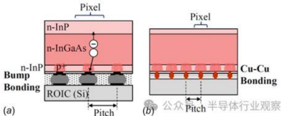
图16：使用 InP/InGaAs/InP 光电二极管通过像素级集成与硅芯片中的读出电路键合的短波长红外传感器：
