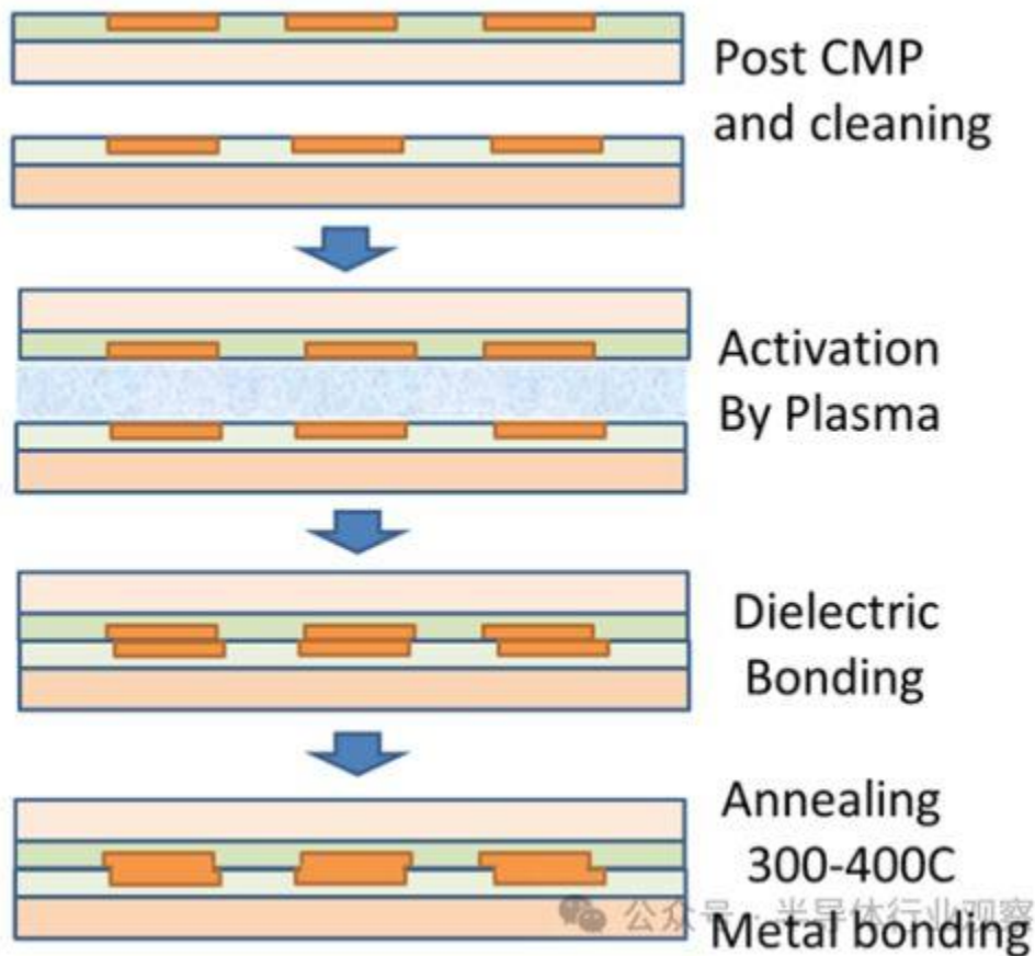
图18：直接键合互联的工艺流程
