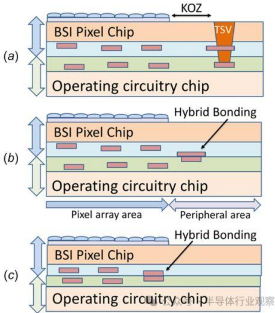
图8：芯片间键合和互连方法，其中（a）直接电介质键合，然后采用用于芯片间互连的后通孔 TSV，（b）外围区域的混合键合，以及（c）像素阵列下的混合键合
