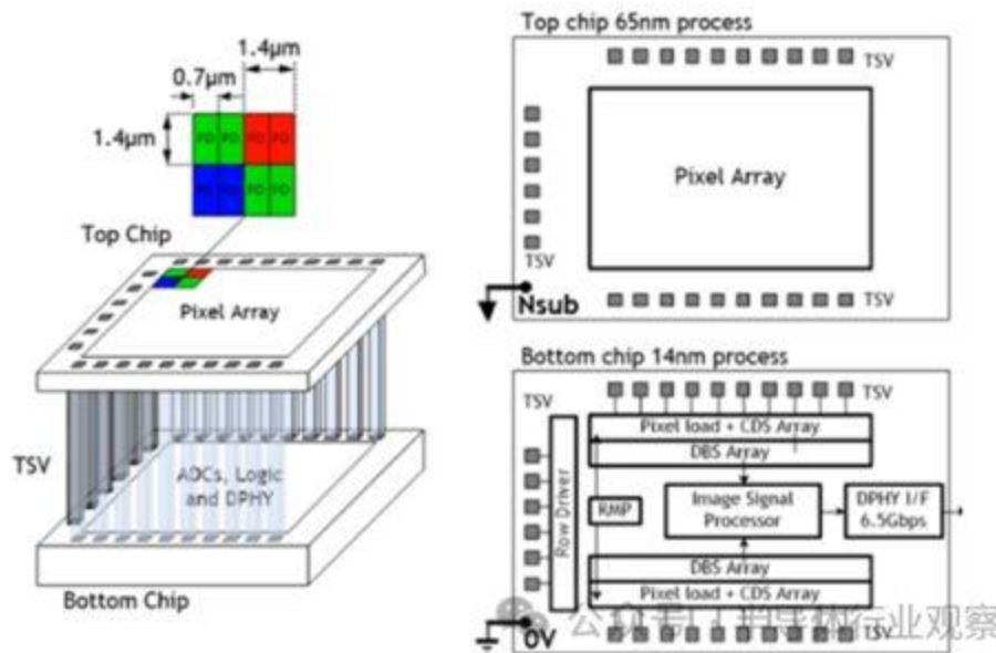
图7：采用 65 nm/14 nm 技术处理的双光电二极管堆叠芯片 BSI-CIS
