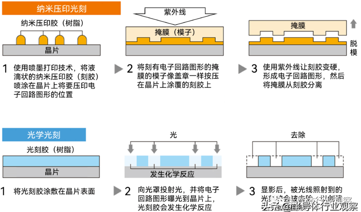
紫外纳米压印光刻与光学光刻流程对比 (图源：果壳硬科技)
