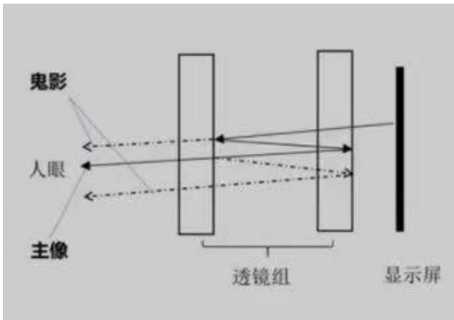
图表17：鬼影降低画面对比度
