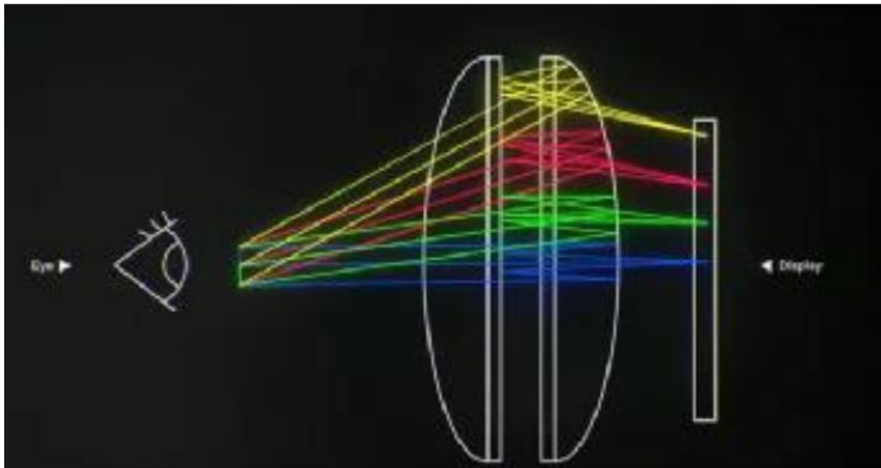
图表14：两片式折叠光路
