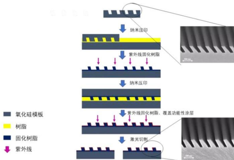
图表43：表面浮雕光栅大批量复制量产工艺
