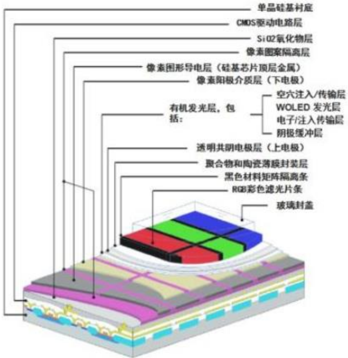
图表21：Micro OLED原理图
