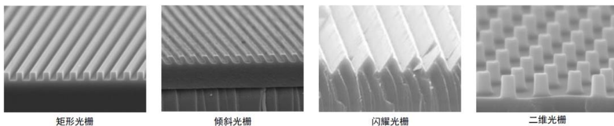
图表37：表面浮雕光栅种类
