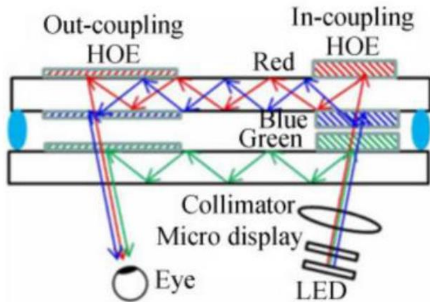
图表49：双层体全息光波导原理图
