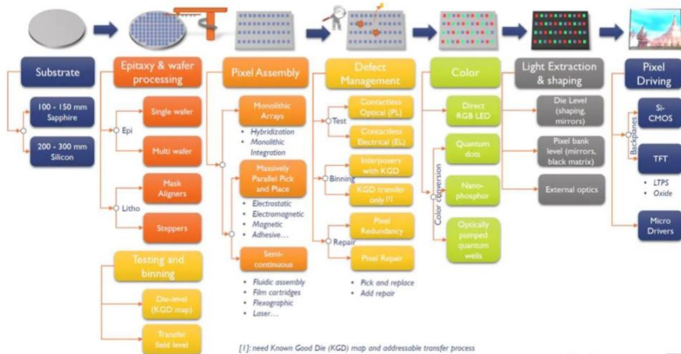
图表56: Micro LED制作工艺
