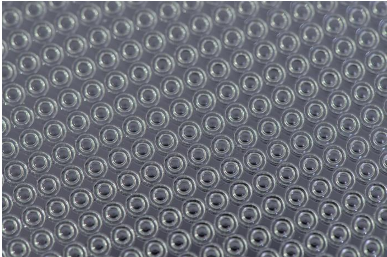
▲ 사진설명: EVG®770 NT 스텝-앤드-리피트 NIL 시스템을 이용해 생산된 웨이퍼 레벨 광학소자용 300mm 스텝 앤 리피트 마스터의 확대 이미지
